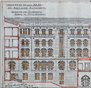
Los planos permiten reconstruir la larga y compleja historia de la iglesia.
